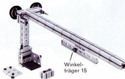
73.3 Träger Baustufe 1
