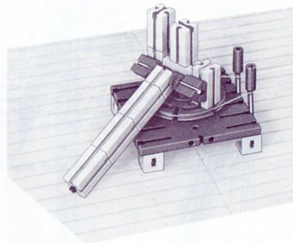
47.5 Baustufe 5
