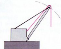
29.3 Einziehausleger
