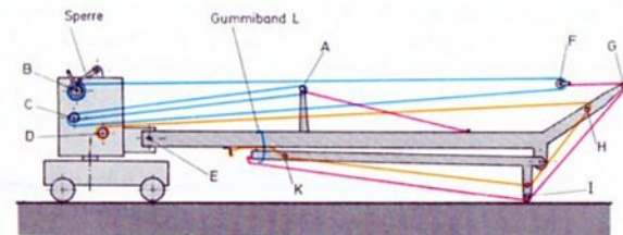
54.1 Seilführung
