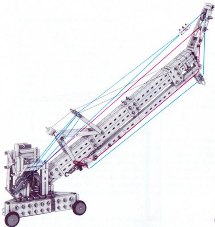
54.3 Aufrichten I
