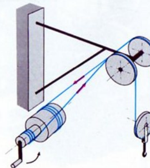
17.2 Wandkran mit Differentialflaschenzug
