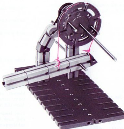
25.2 Baustufe 2 (Bandbremse)
