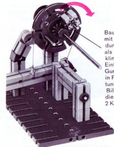
25.3 Baustufe 3 (1 Klinke)
