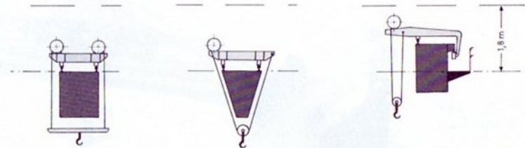
71.4 obenliegende Katze
