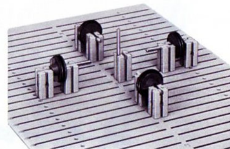
9.4 Baustufe zu 9.3
