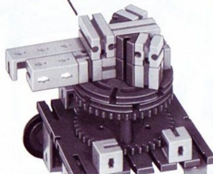
60.3 Baustufe 3
