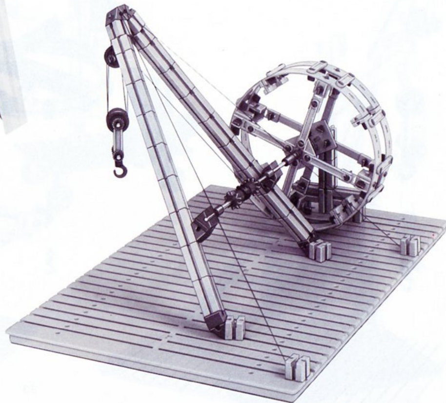
10.2 Baustufe 1
