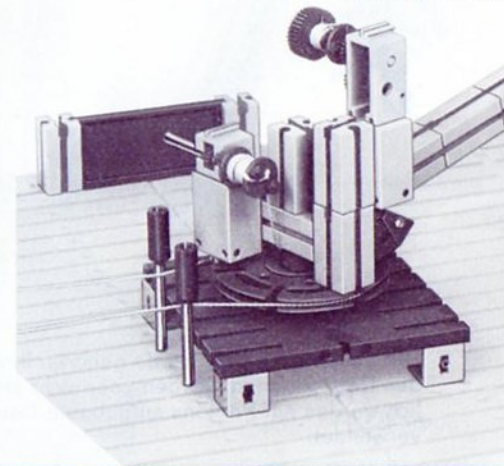
47.5 Baustufe 5
