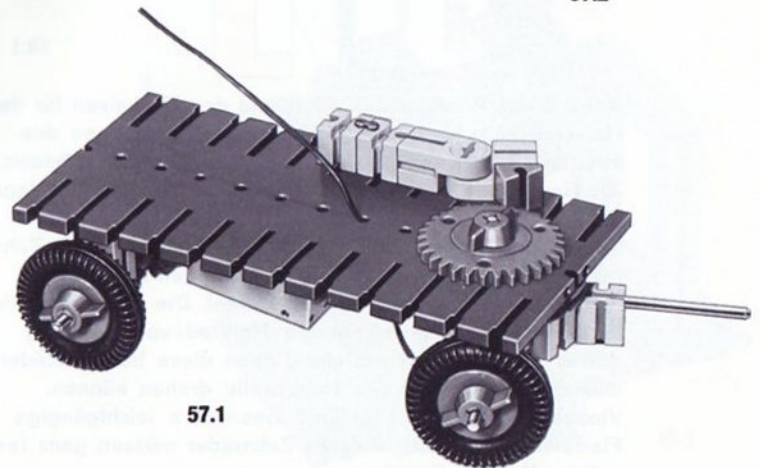
ohne Differential
